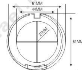
ES1014A-4 SIZE: \varnothing 61 \times H20.5\text{mm}
