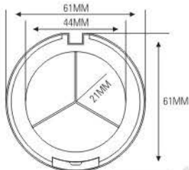
ES1014A-3 SIZE: \varnothing 61 \times H20.5\text{mm}
