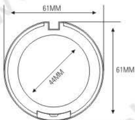
ES1014A-1 SIZE: \varnothing 61 \times H20.5\text{mm}
